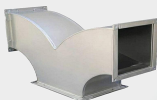
Ống gió Rẽ nhánh Drop Cheek Breechers
